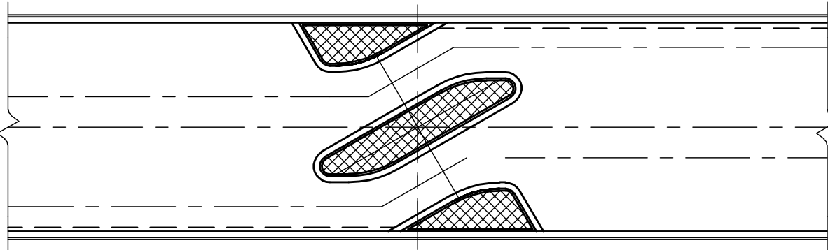
TWO LANE ANGLED - 10m + C/WAY N.T.S.
