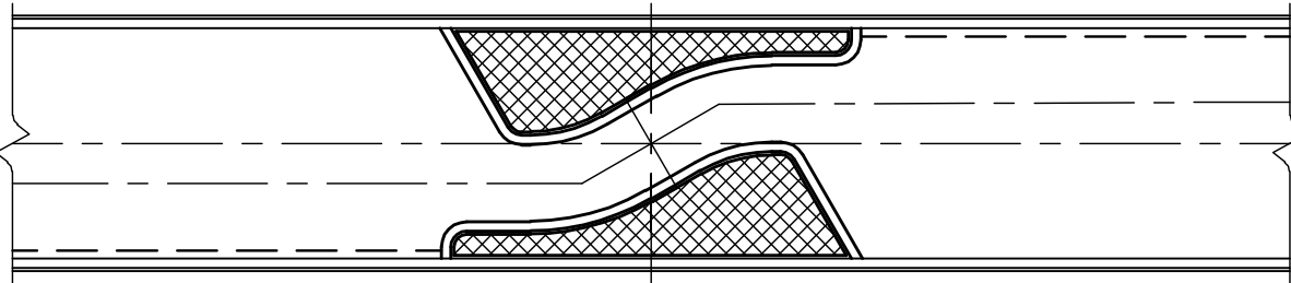
SINGLE LANE ANGLED - 8m C/WAY N.T.S.
