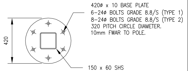
POLE BASEPLATE
